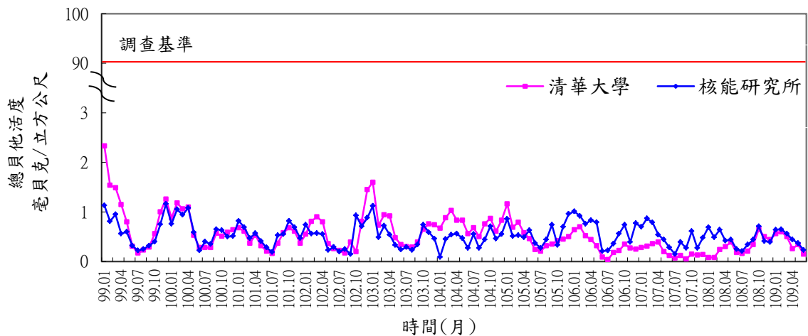
附圖 3.3 核能研究所及清華大學環境空浮微粒試樣總貝他平均活度變動圖
