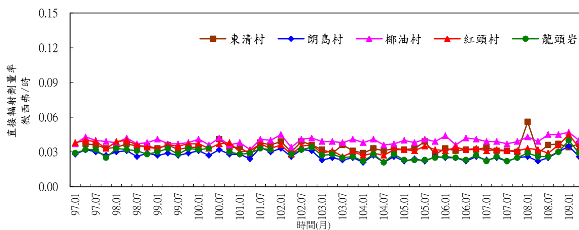
附圖 4.1 蘭嶼地區環境直接輻射劑量率變動圖(TLD)
