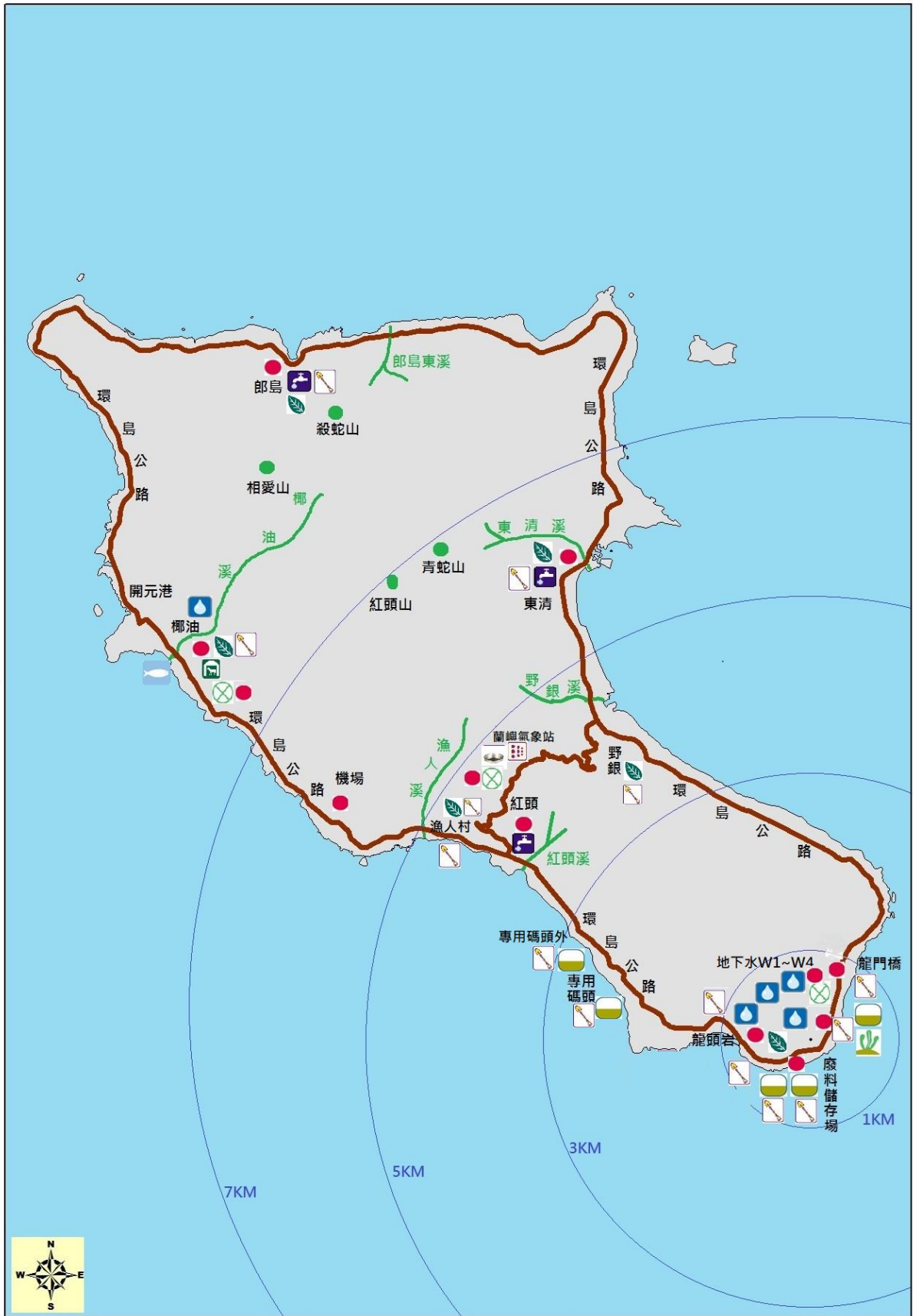
附圖 1.9 蘭嶼低放貯存場環境輻射監測取樣位置圖
