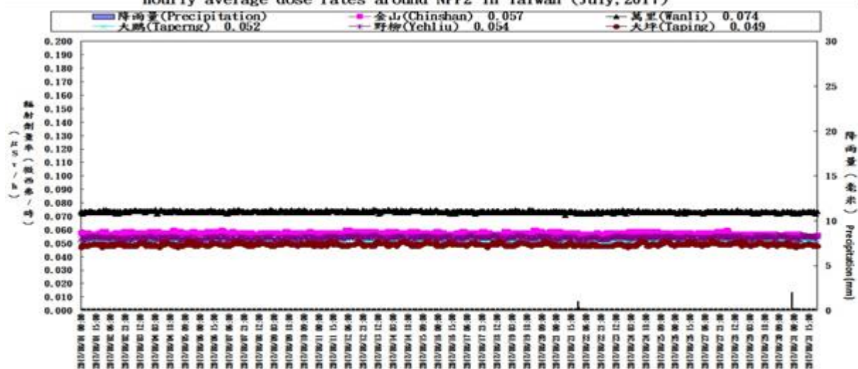
核二廠輻安預警自動監測時平均劑量率(中華民國一百零六年八月) Hourly average dose rates around NPP2 in Taiwan (Aug, 2017)
