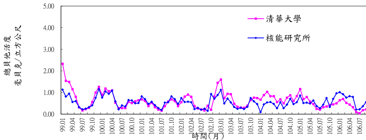
附圖 3.3 研究用核設施環境空浮微粒試樣總貝他平均活度變動圖
