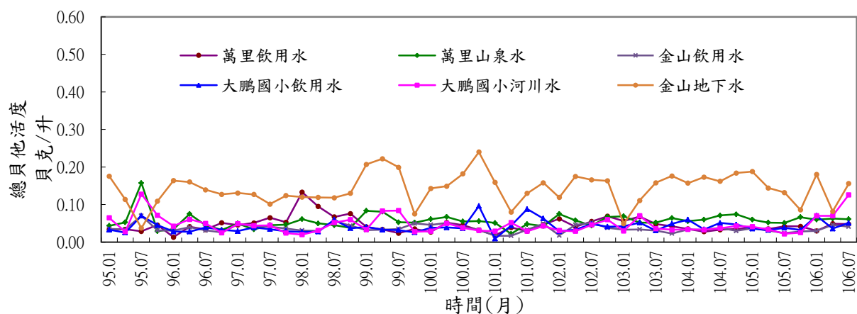
附圖 2.8 核二廠環境水樣總貝他活度變動圖
