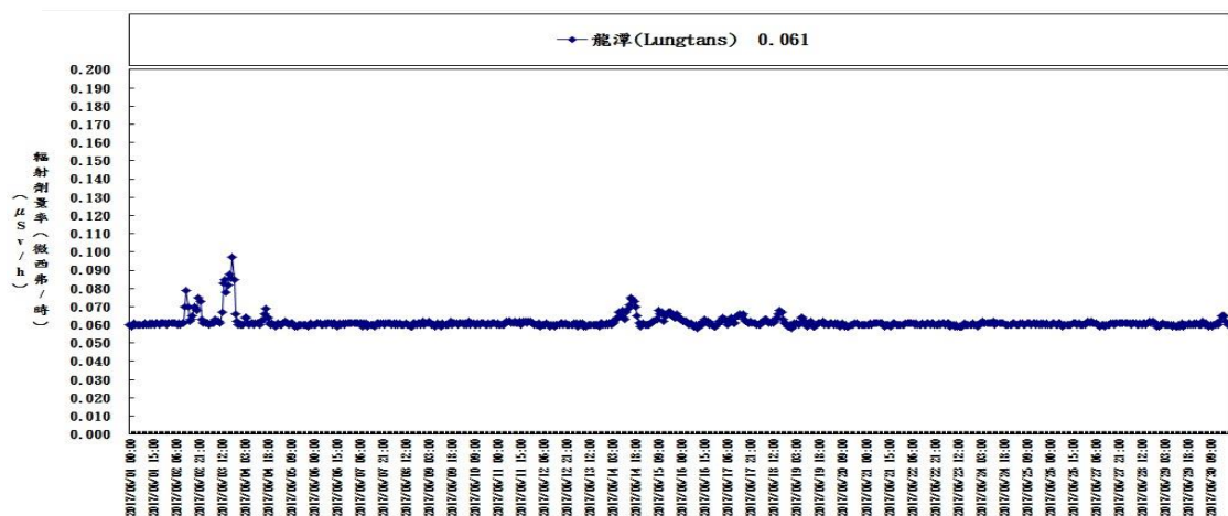
核能研究所地區輻安預警自動監測時平均劑量率(中華民國一百零六年六月) Hourly average dose rates around INER in Taiwan (June, 2017)
