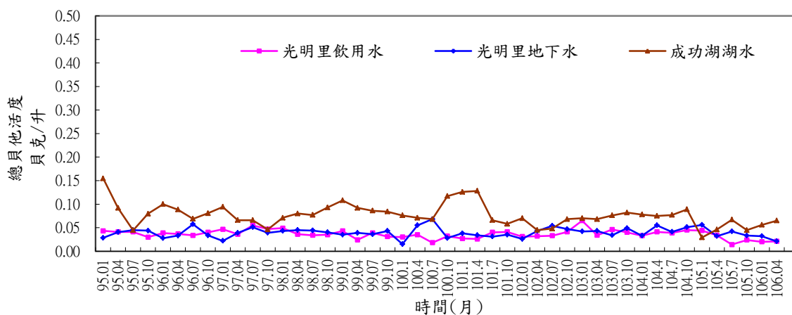
附圖3.5 清華大學環境水樣總貝他活度變動圖
