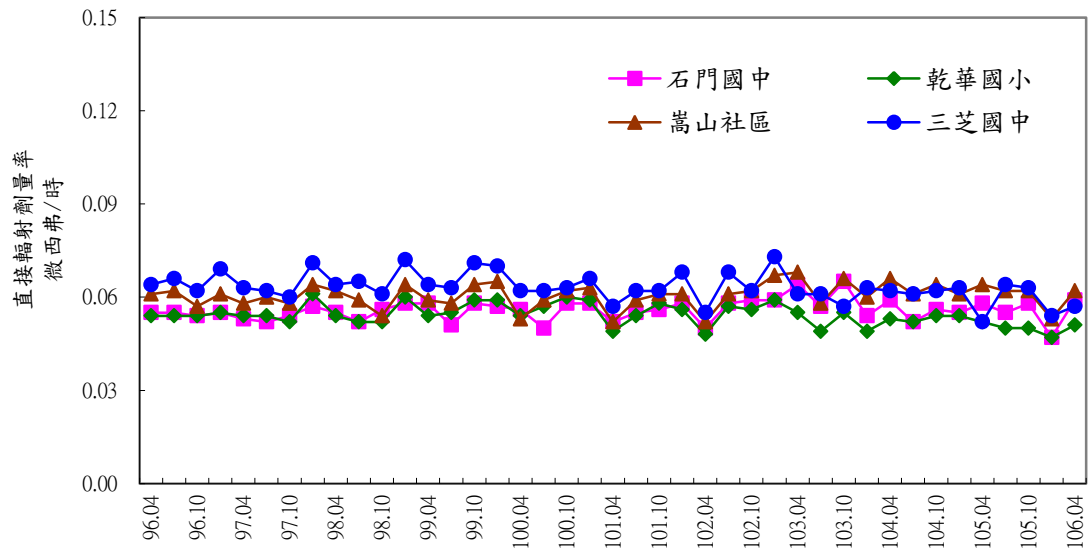
附圖 2.1 核一廠環境直接輻射季平均劑量率變動圖
