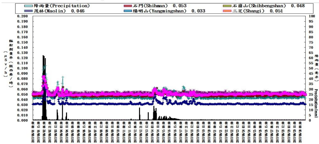
核一廠輻安預警自動監測時平均劑量率(中華民國一百零六年六月)
