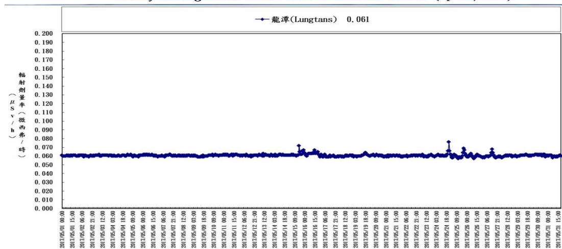
核能研究所地區輻安預警自動監測時平均劑量率(中華民國一百零六年五月) Hourly average dose rates around INER in Taiwan (May, 2017)
