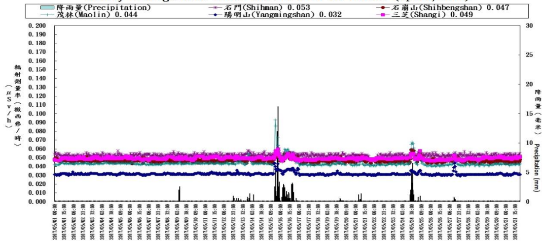
核一廠輻安預警自動監測時平均劑量率(中華民國一百零六年五月)
