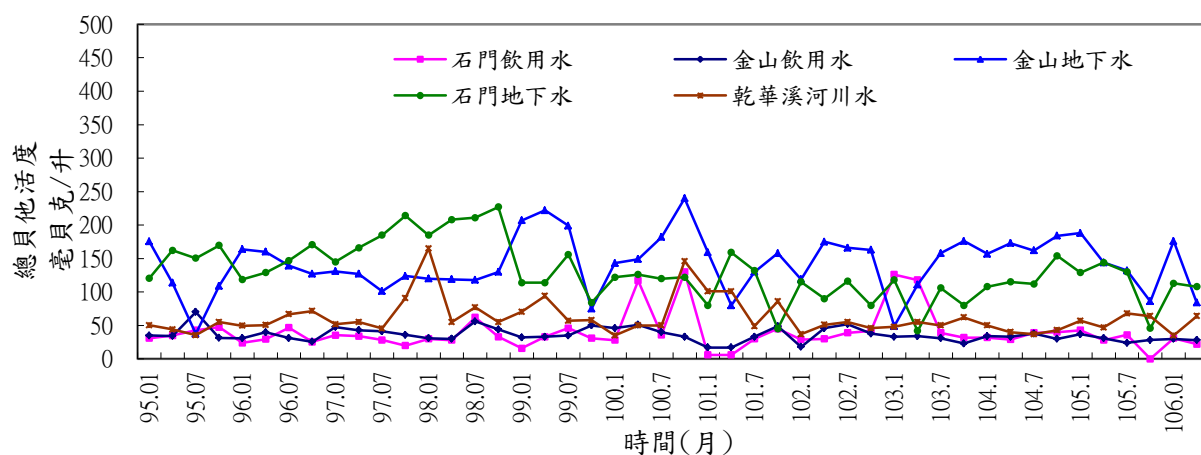
附圖 2.7 核一廠環境水樣總貝他活度變動圖
