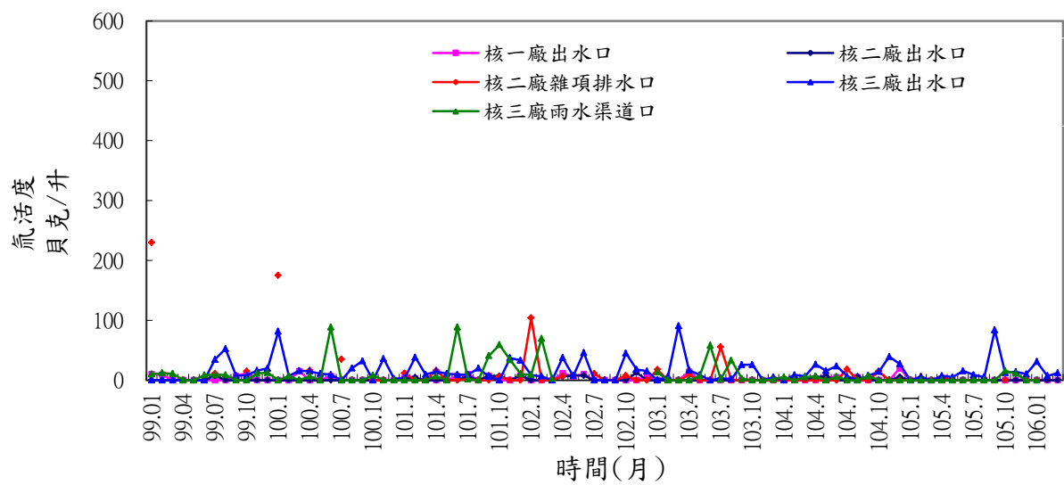
附圖 2.10 核電廠排放口水樣氣活度變動圖
