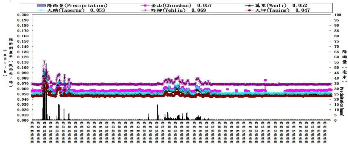
核二廠輻安預警自動監測時平均劑量率(中華民國一百零六年六月) Hourly average dose rates around NPP2 in Taiwan (June, 2017)
