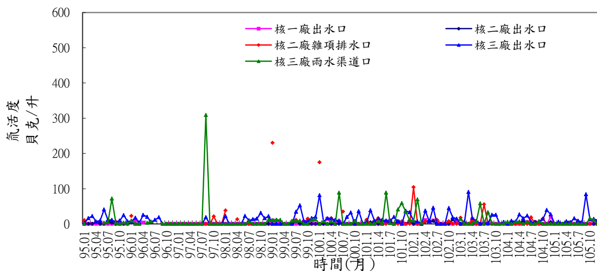
附圖 2.10 核電廠排放口水樣β活度變動圖
