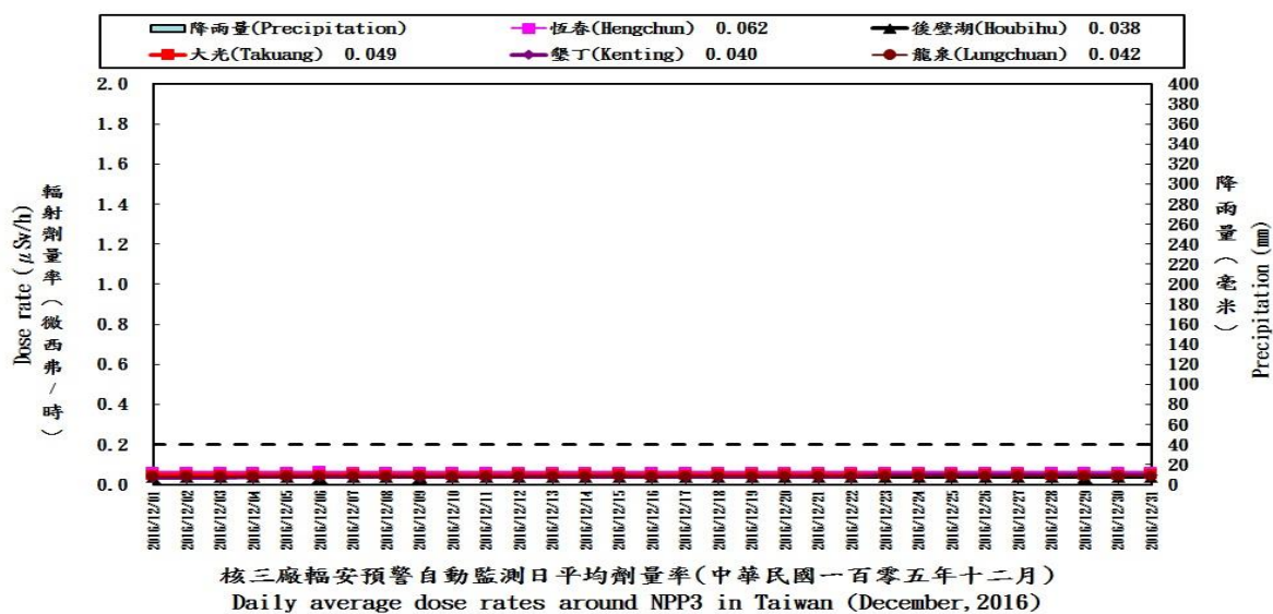
附圖 5.3 核三廠環境輻安預警自動監測日平均劑量率變動圖
