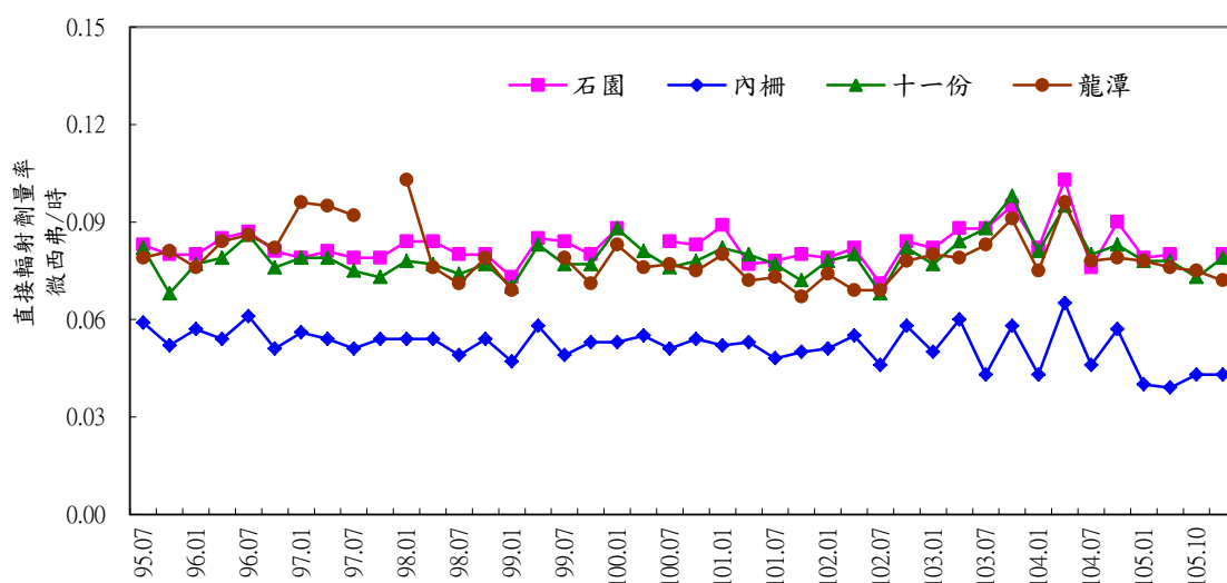
附圖 3.1 核能研究所環境主要方位熱發光劑量計季平均劑量率變動圖
