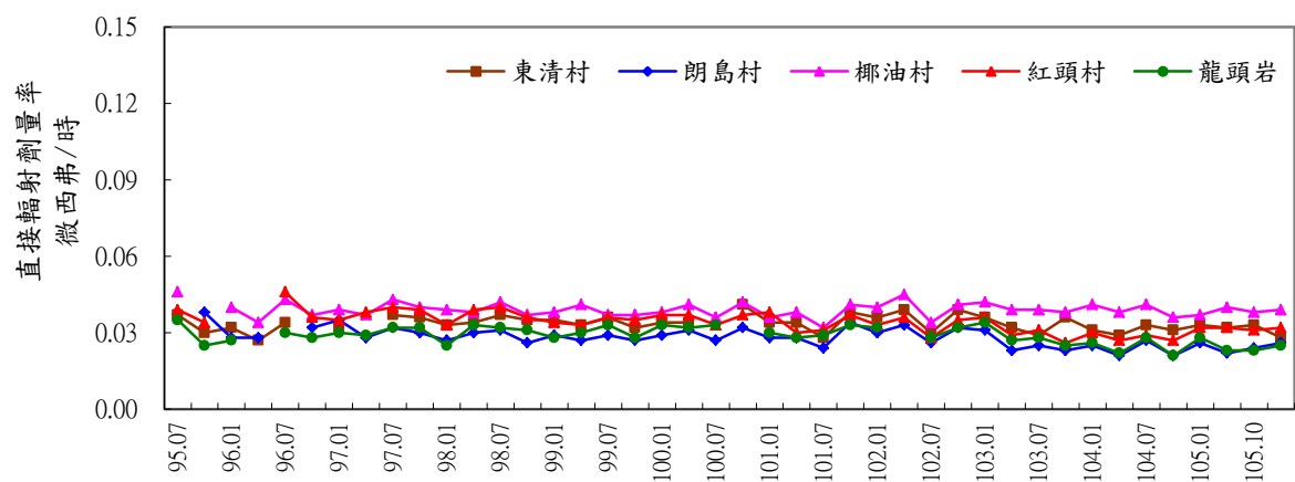
附圖 4.1 蘭嶼貯存場環境主要方位熱發光劑量計季平均劑量率變動圖
