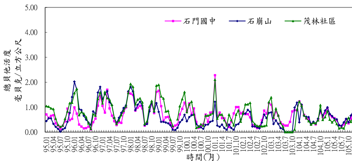
附圖 2.4 核一廠環境空浮微粒試樣總貝他平均活度變動圖
