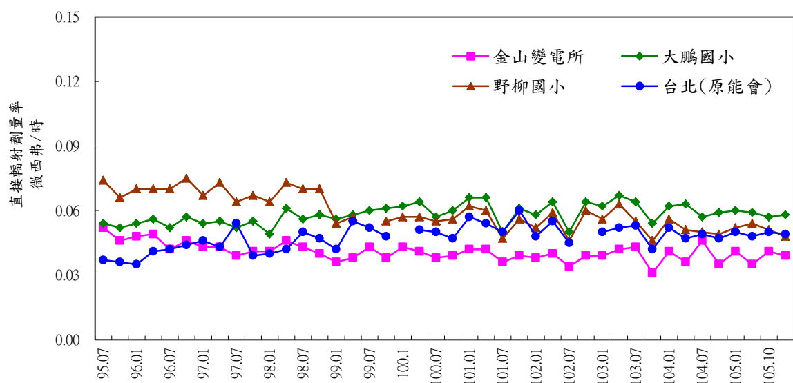
附圖 2.2 核二廠環境主要方位熱發光劑量計季平均劑量率變動圖
