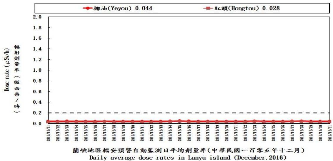
附圖 5.5 蘭嶼地區環境輻安預警自動監測日平均劑量率變動圖
