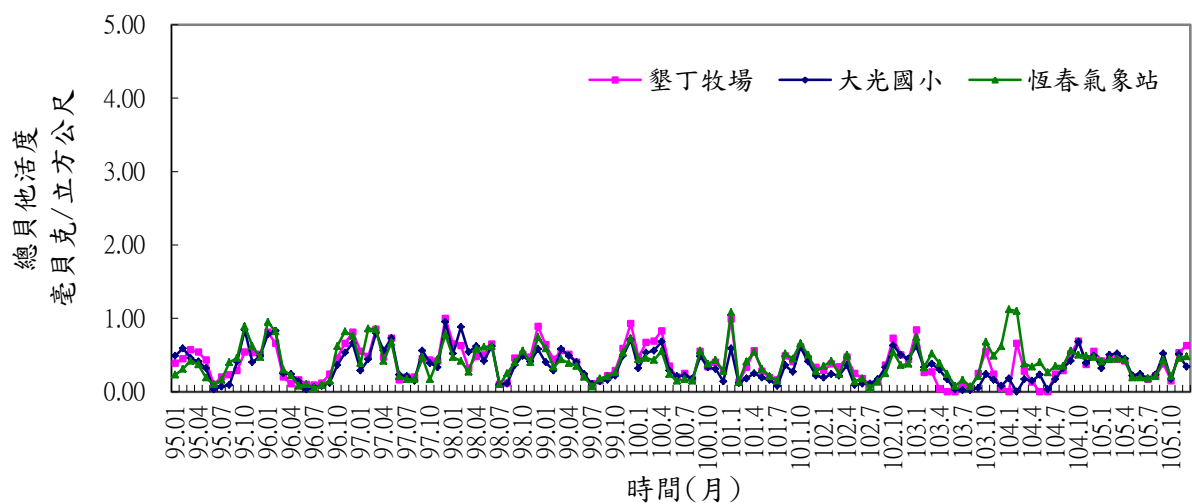
附圖 2.6 核三廠環境空浮微粒試樣總貝他平均活度變動圖
