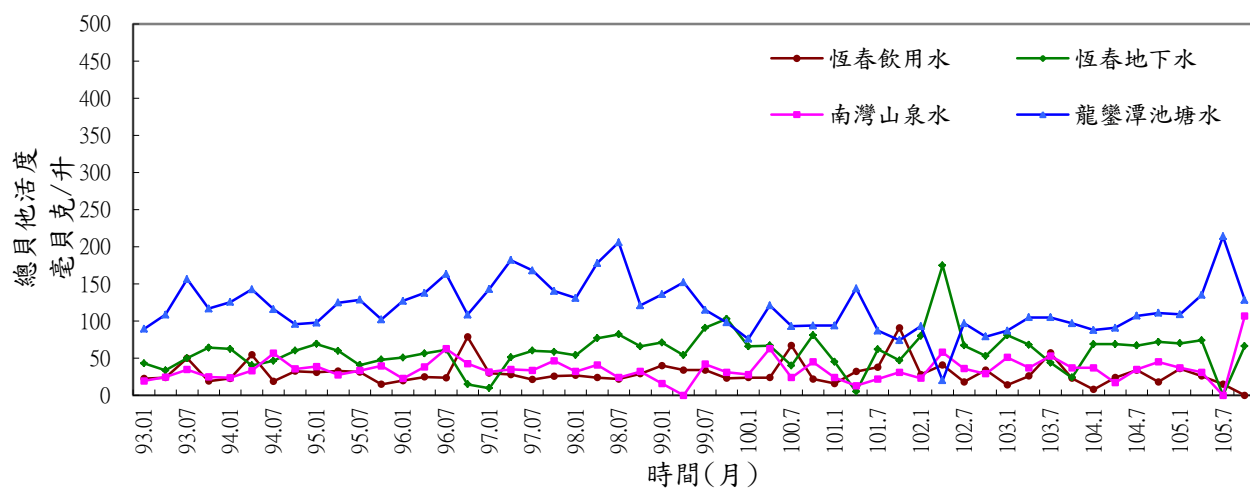
附圖 2.9 核三廠環境水樣總貝他活度變動圖
