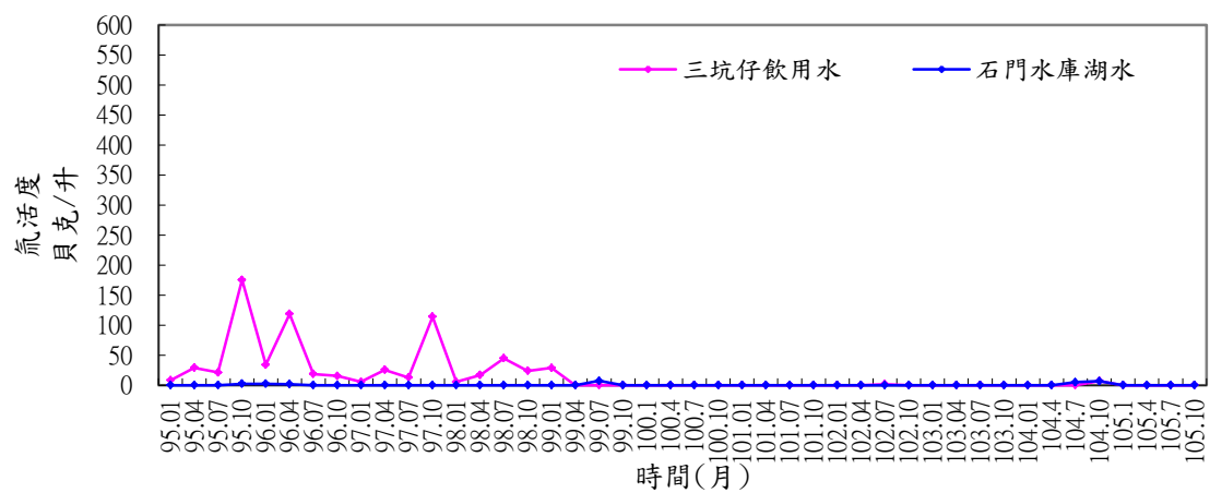
附圖3.6 核能研究所環境水樣氡活度變動圖
