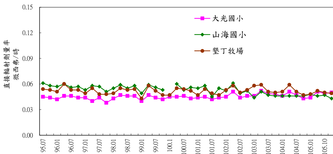
附圖 2.3 核三廠環境主要方位熱發光劑量計季平均劑量率變動圖
