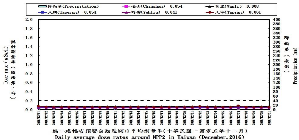
附圖 5.2 核二廠環境輻安預警自動監測日平均劑量率變動圖
