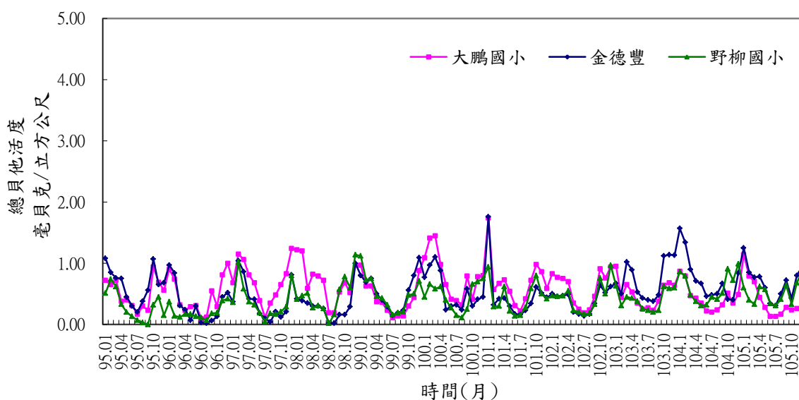
附圖 2.5 核二廠環境空浮微粒試樣總貝他平均活度變動圖
