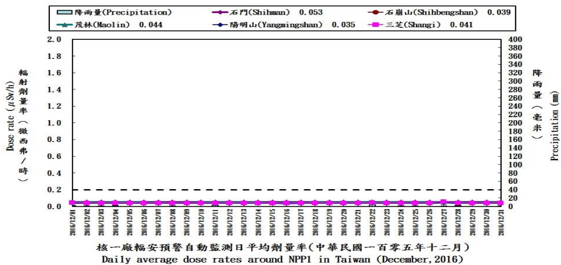
附圖 5.1 核一廠環境輻安預警自動監測日平均劑量率變動圖
