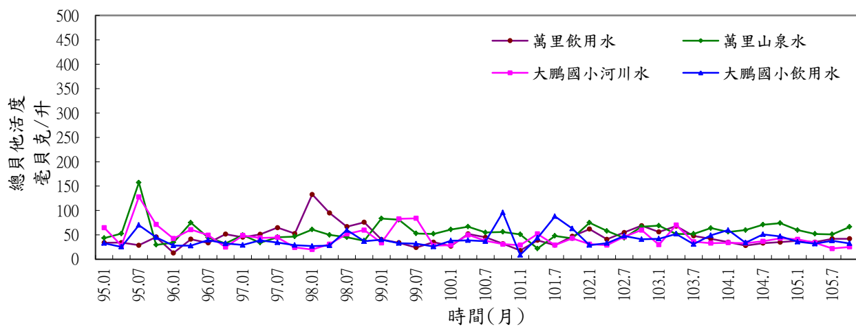
附圖 2.8 核二廠環境水樣總貝他活度變動圖
