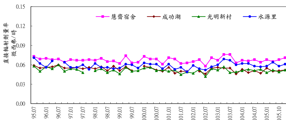
附圖 3.2 清華大學環境主要方位熱發光劑量計季平均劑量率變動圖
