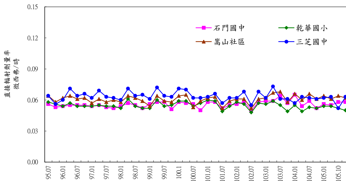
附圖 2.1 核一廠環境主要方位熱發光劑量計季平均劑量率變動圖
