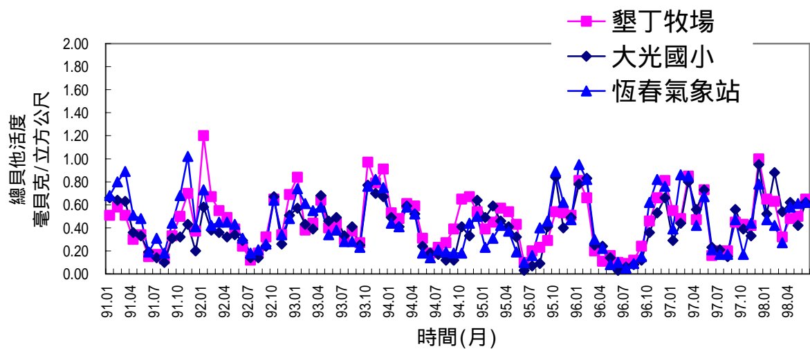
圖 2.9 核能三廠環境空浮微粒試樣總貝他平均活度變動圖
