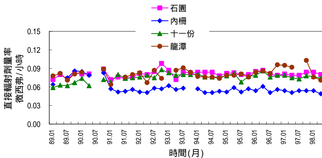
圖 2.15 核能研究所環境主要方位熱發光劑量計季平均劑量率變動圖
