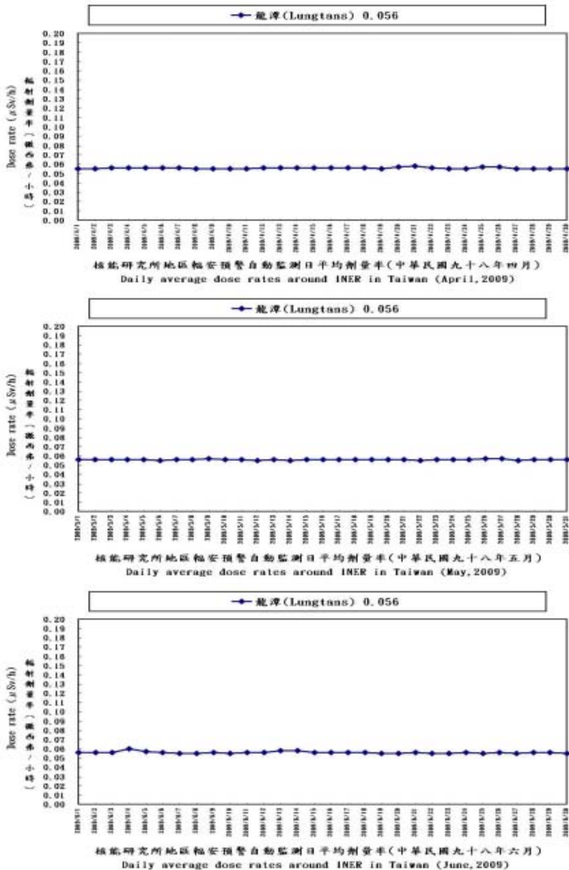
圖 2.14 核能研究所環境輻安預警自動監測日平均劑量率變動圖
