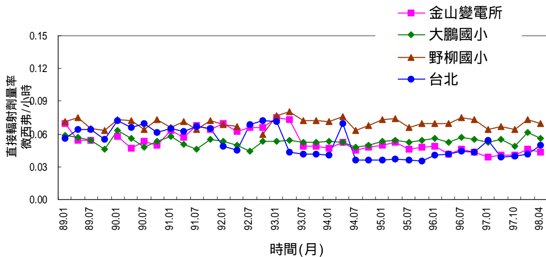
圖 2.5 核能二廠環境主要方位熱發光劑量計季平均劑量率變動圖
