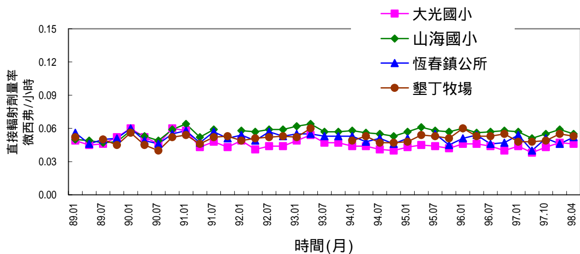
圖 2.6 核能三廠環境主要方位熱發光劑量計季平均劑量率變動圖
