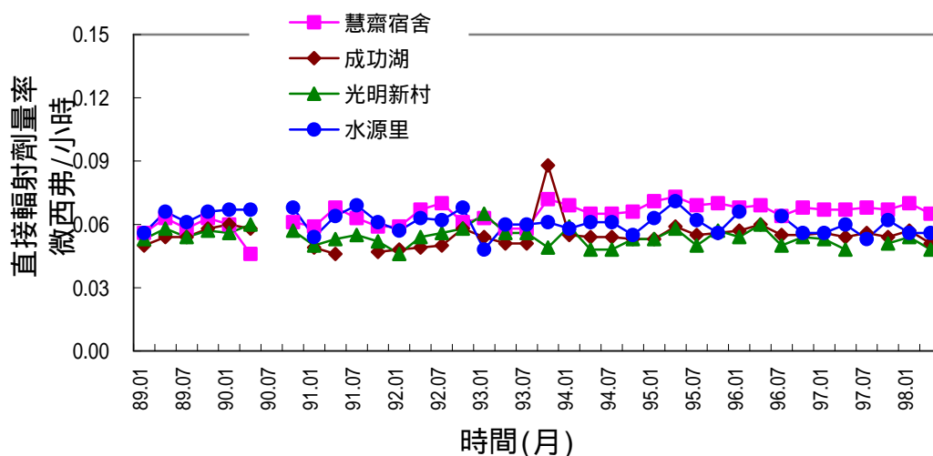
圖 2.16 清華大學環境主要方位熱發光劑量計季平均劑量率變動圖
