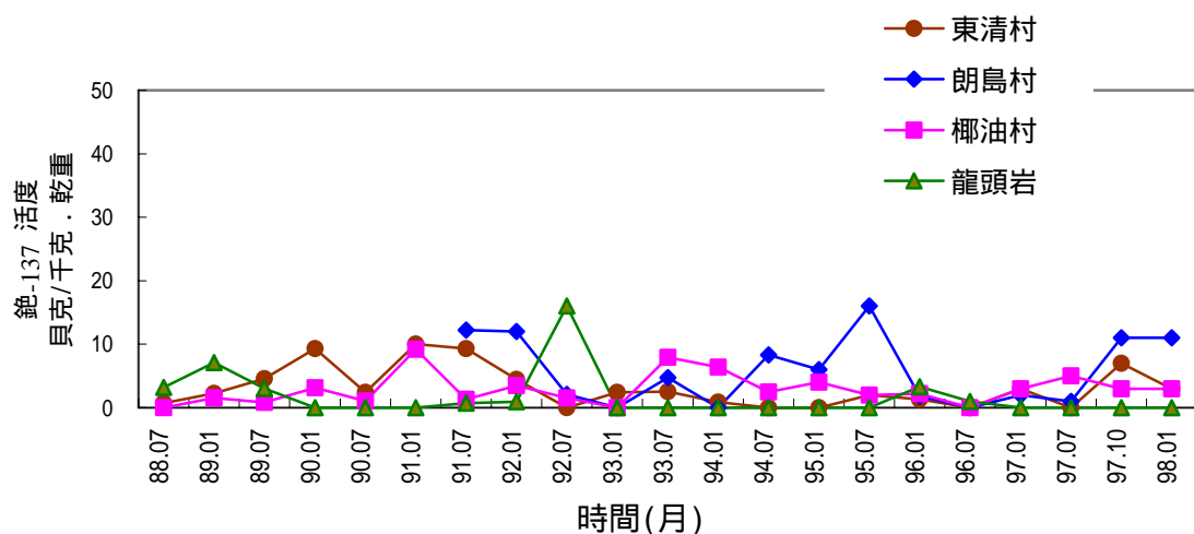
圖 2.23 蘭嶼地區環境土壤試樣加馬能譜分析銫-137 活度變動圖
