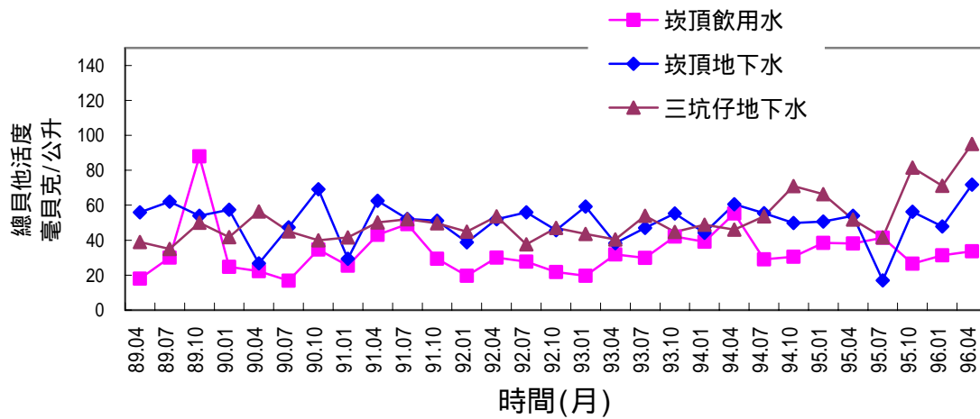
圖2.19 核能研究所環境水樣總貝他活度變動圖
