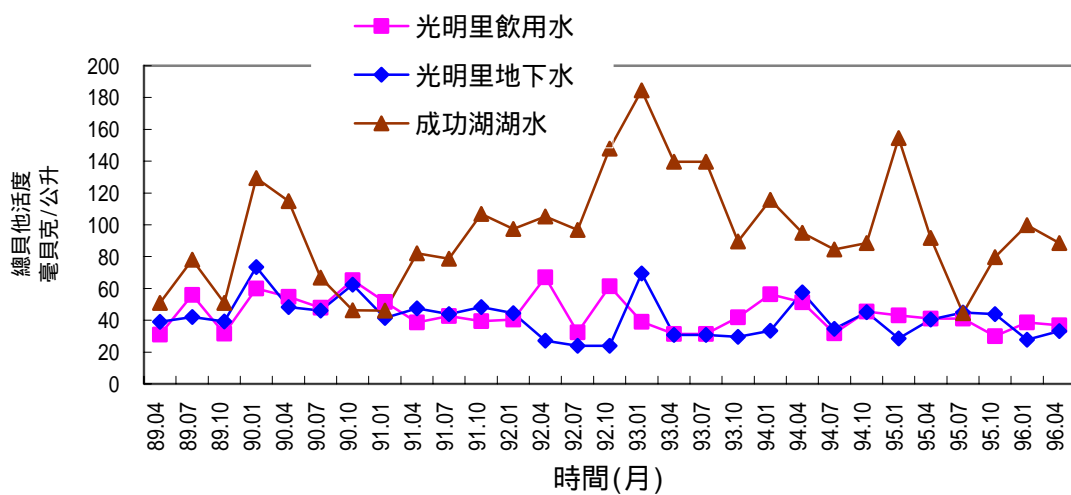
圖2.20 清華大學環境水樣總貝他活度變動圖
