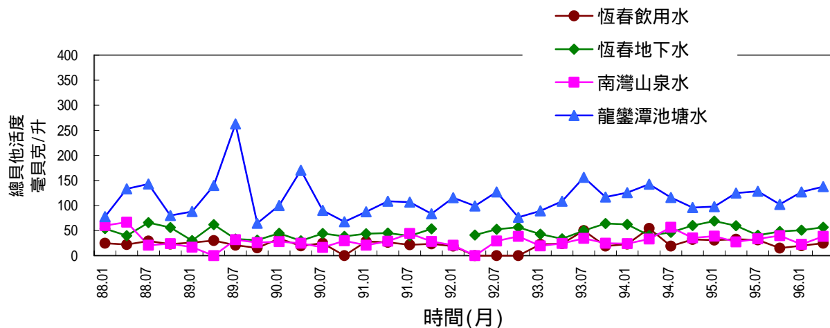
圖 2.12 核能三廠環境水樣總貝他活度變動圖
