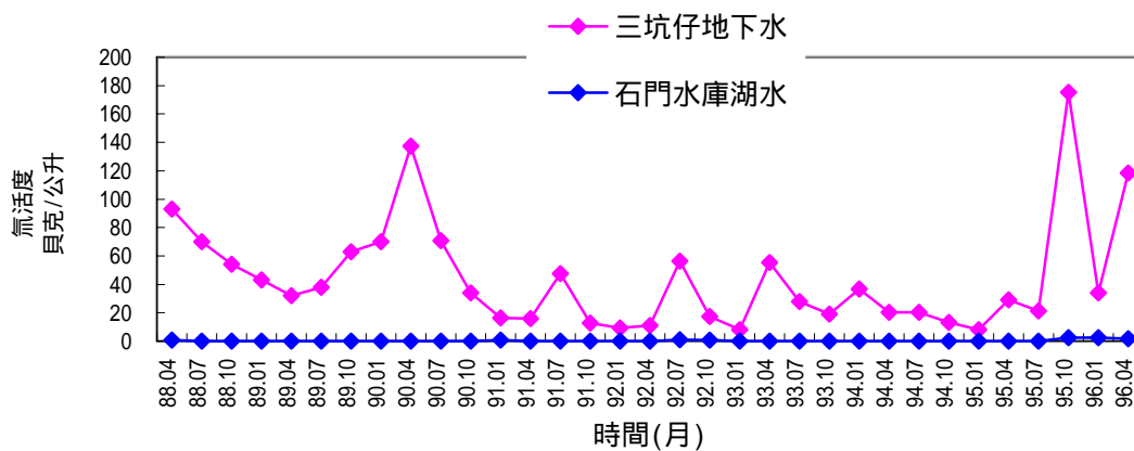
圖2.21 核能研究所環境水樣氚活度變動圖
