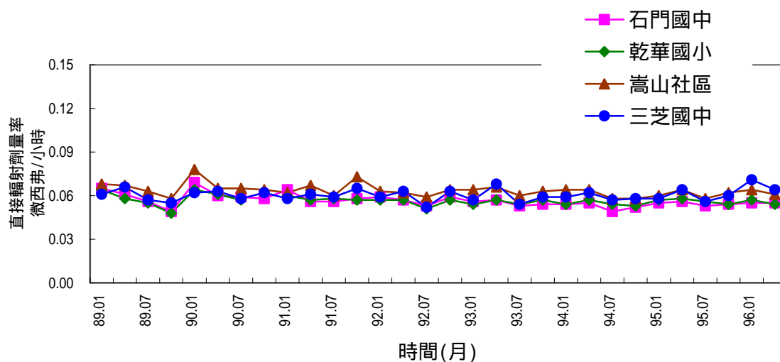
圖 2.4 核能一廠主要方位熱發光劑量計季平均劑量率變動圖
