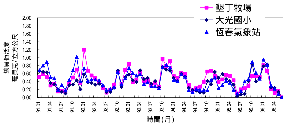
圖 2.9 核能三廠空浮微粒總貝他平均活度變動圖 表 2.16 核能電廠空浮微粒總貝他活度分析結果(抽氣法)
