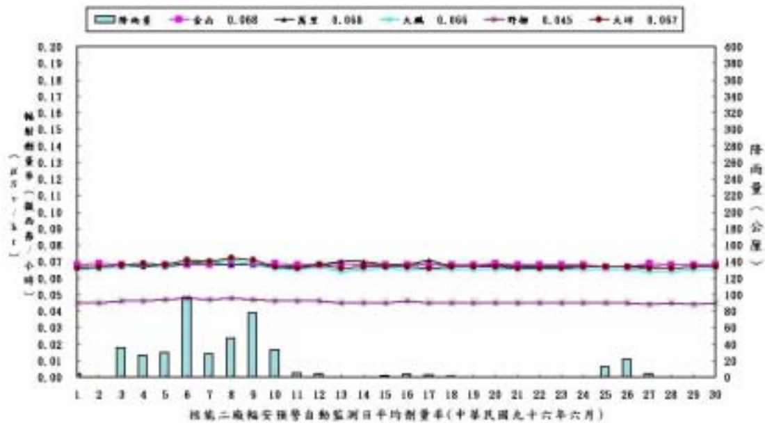
圖 2.2 核能二廠輻安預警自動監測日平均劑量率變動圖
