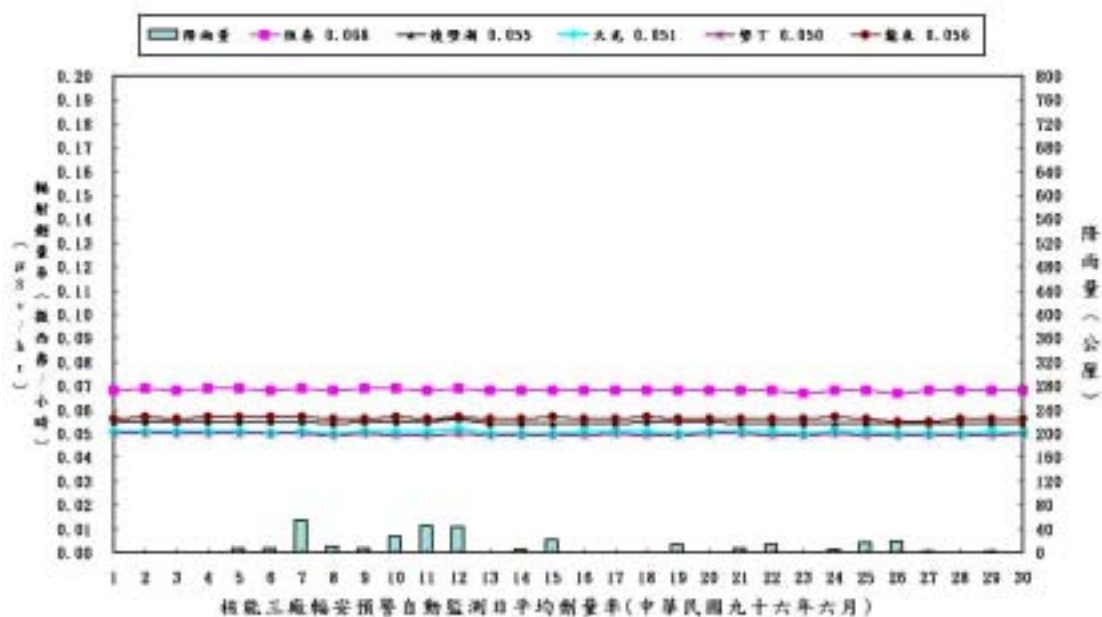
圖 2.3 核能三廠輻安預警自動監測日平均劑量率變動圖
