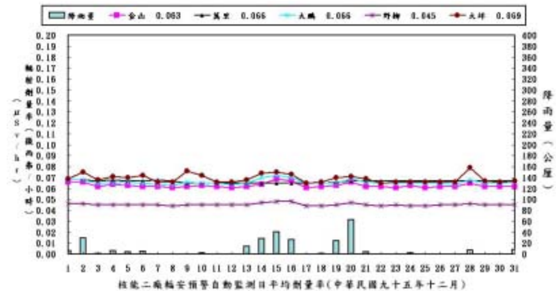
圖 2.2 核能二廠輻安預警自動監測日平均劑量率變動圖
