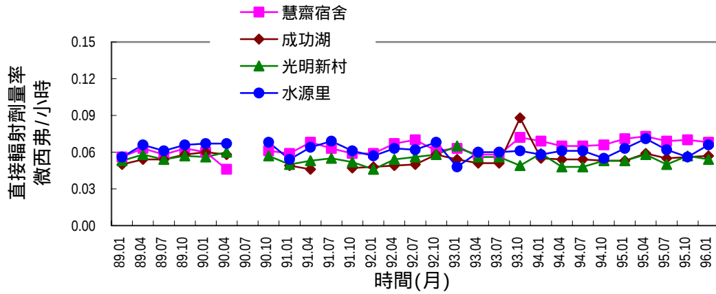
圖 2.16 清華大學主要方位熱發光劑量計季平均劑量率變動圖
