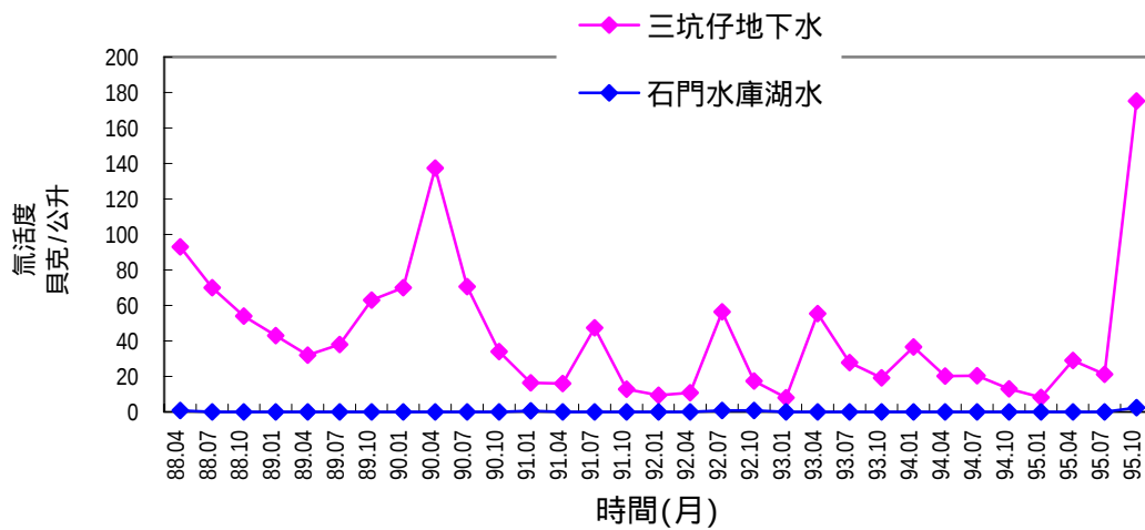
圖2.21 核能研究所環境水樣氚活度變動圖
