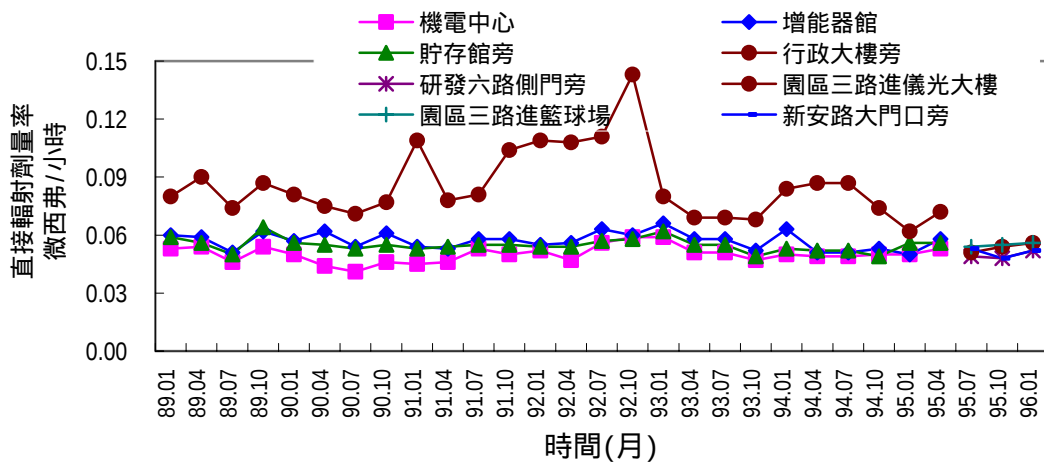
圖 2.17 同步輻射研究中心熱發光劑量計季平均劑量率變動圖
