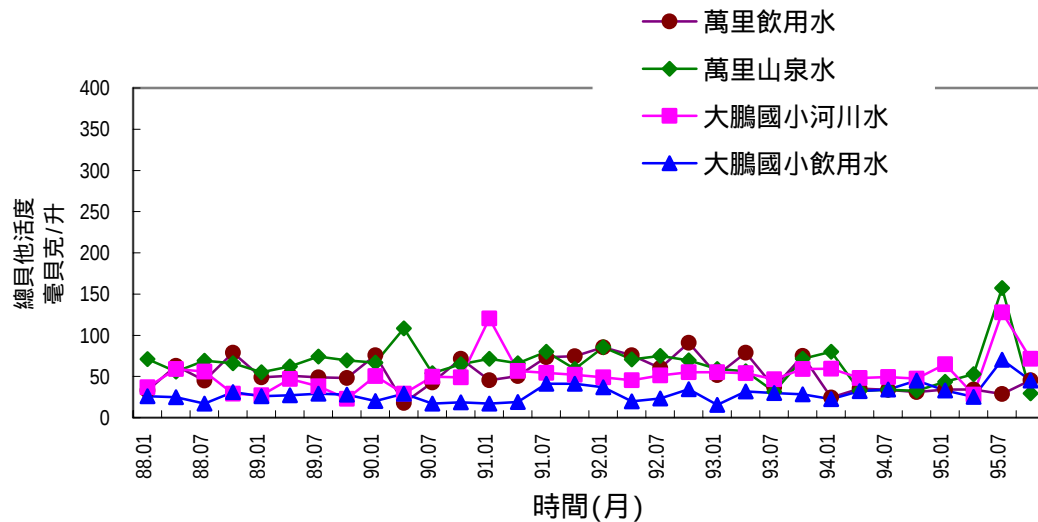
圖 2.11 核能二廠環境水樣總貝他活度變動圖
