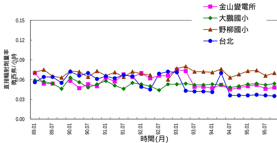
圖 2.5 核能二廠主要方位熱發光劑量計季平均劑量率變動圖
