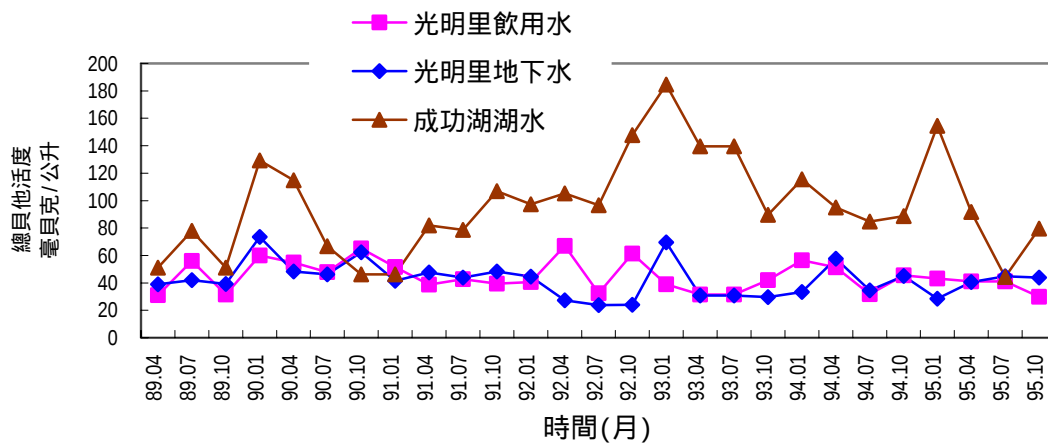
圖2.20 清華大學環境水樣總貝他活度變動圖
