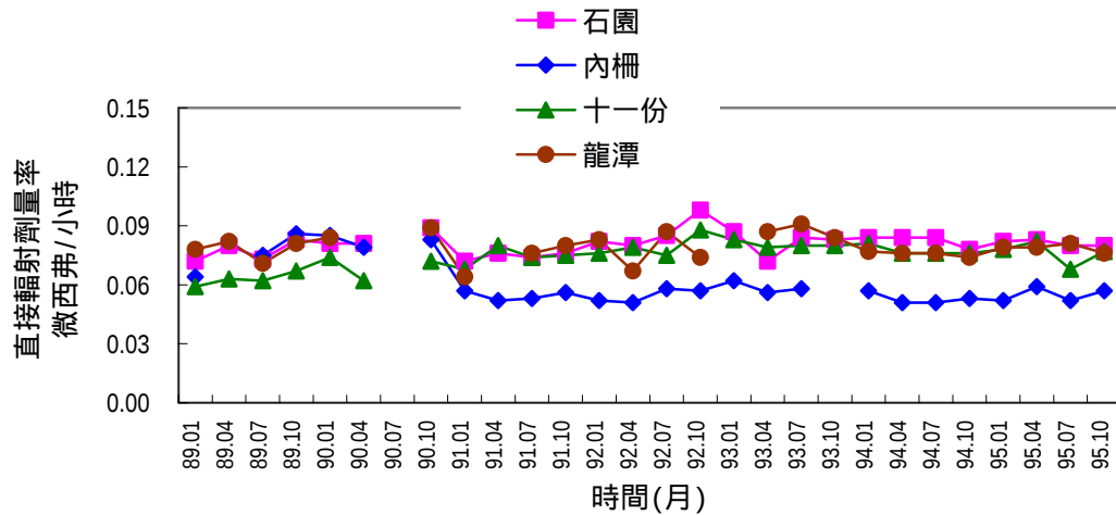
圖 2.15 核能研究所主要方位熱發光劑量計季平均劑量率變動圖
