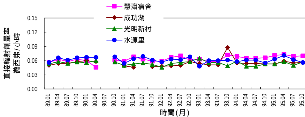
圖 2.15 核能研究所主要方位熱發光劑量計季平均劑量率變動圖
