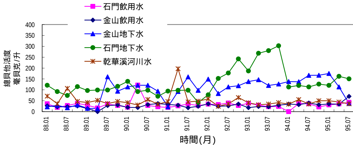
圖 2.10 核能一廠環境水樣總貝他活度變動圖
