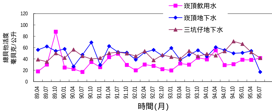
圖2.19 核能研究所環境水樣總貝他活度變動圖
