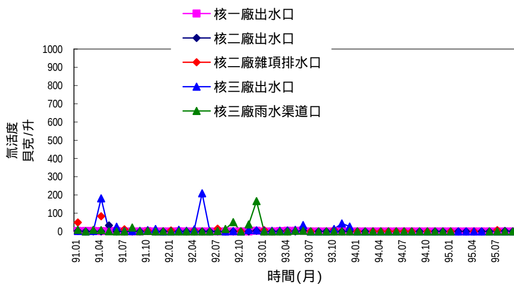
圖 2.13 核能電廠排放口水樣氡活度變動圖
