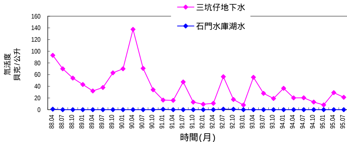
圖 2.21 核能研究所環境水樣氚活度變動圖
