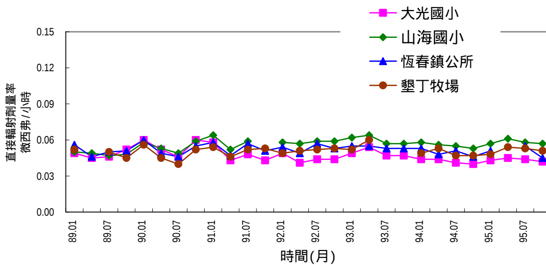
圖 2.6 核能三廠主要方位熱發光劑量計季平均劑量率變動圖
