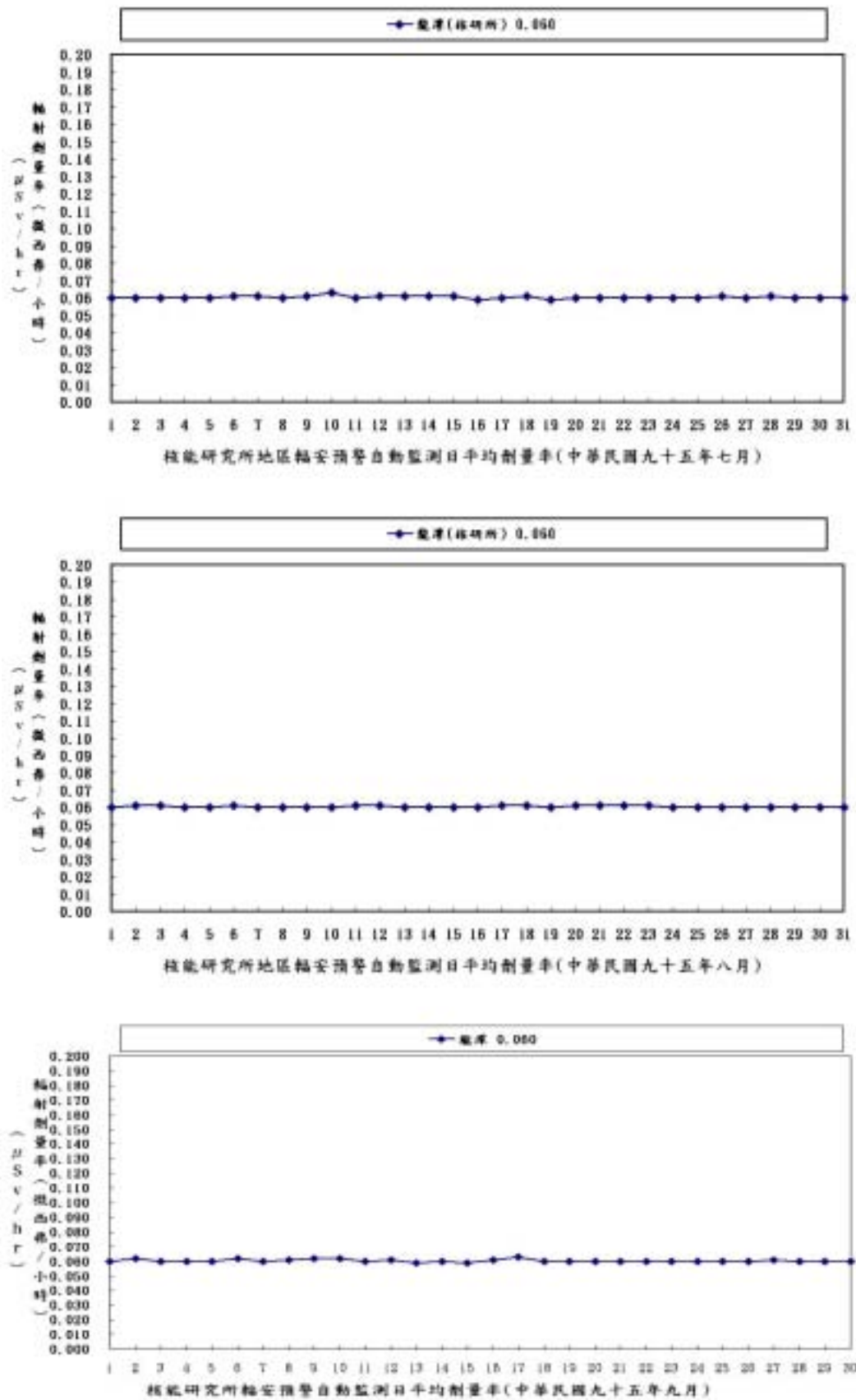
圖 2.14 核能研究所輻安預警自動監測日平均劑量率變動圖
