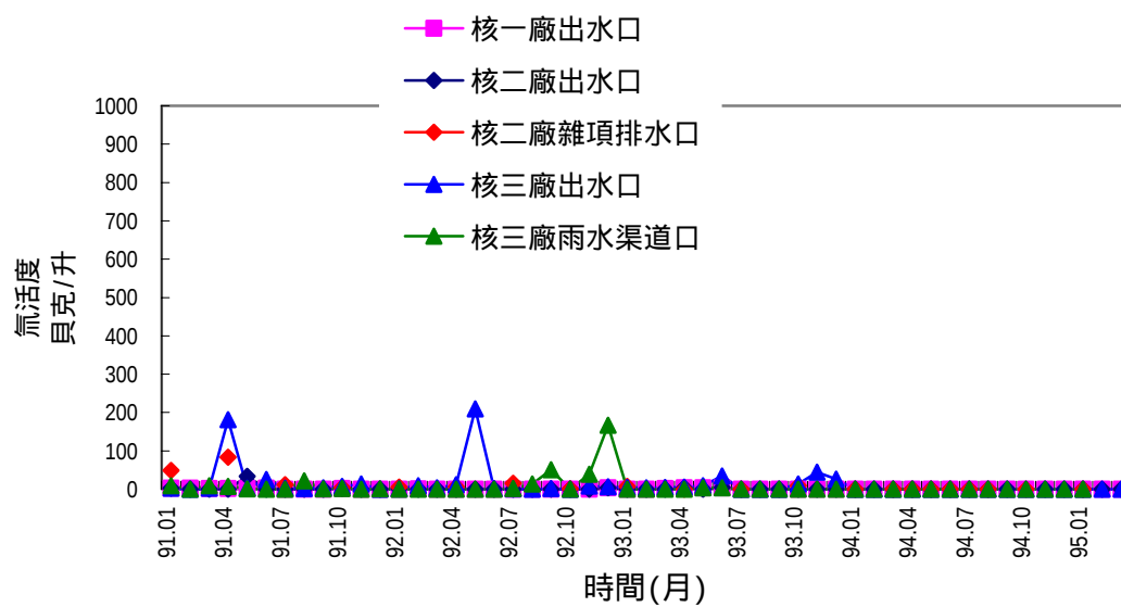
圖 2.13 核能電廠排放口水樣氡活度變動圖
