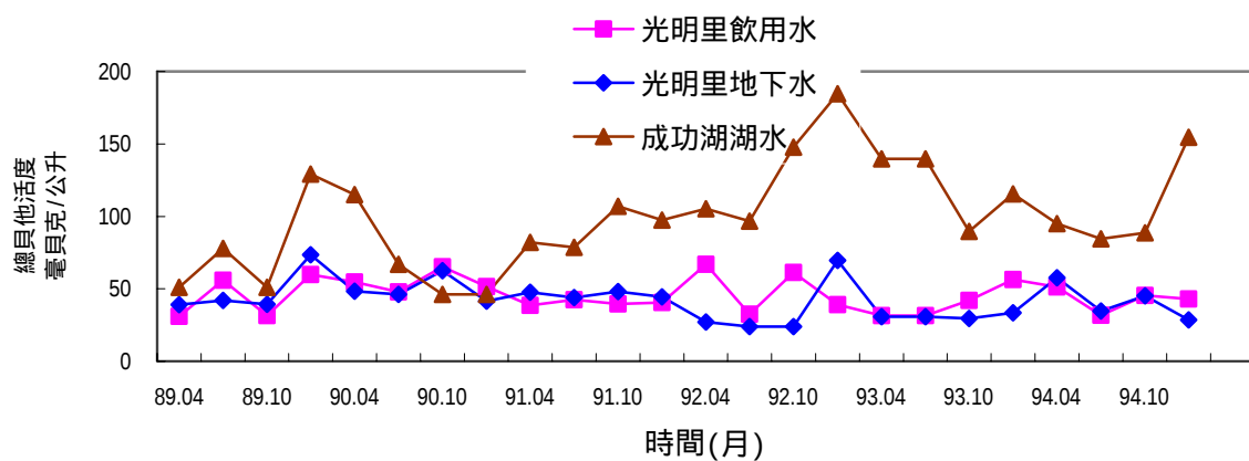
圖2.20 清華大學環境水樣總貝他活度變動圖
