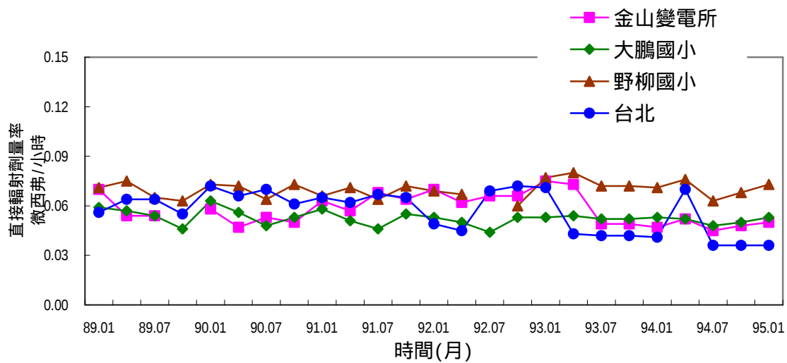
圖 2.5 核能二廠主要方位熱發光劑量計季平均劑量率變動圖
