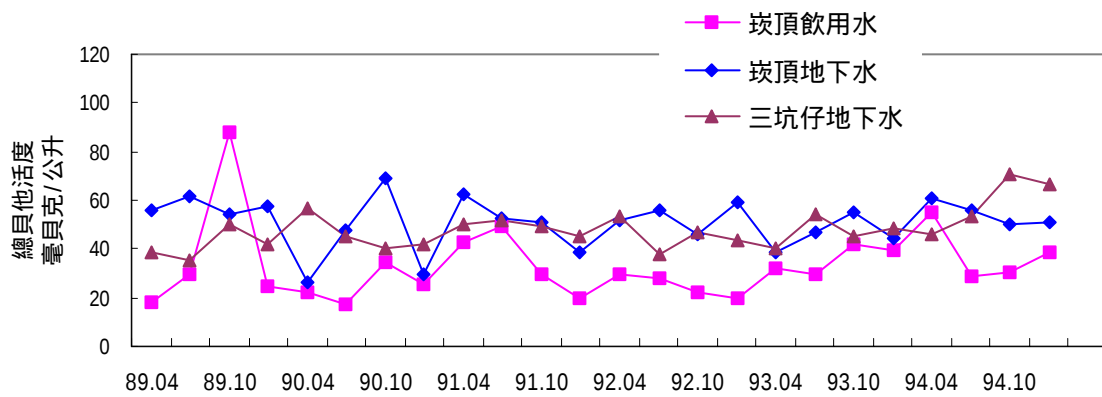
圖2.19 核能研究所環境水樣總貝他活度變動圖
