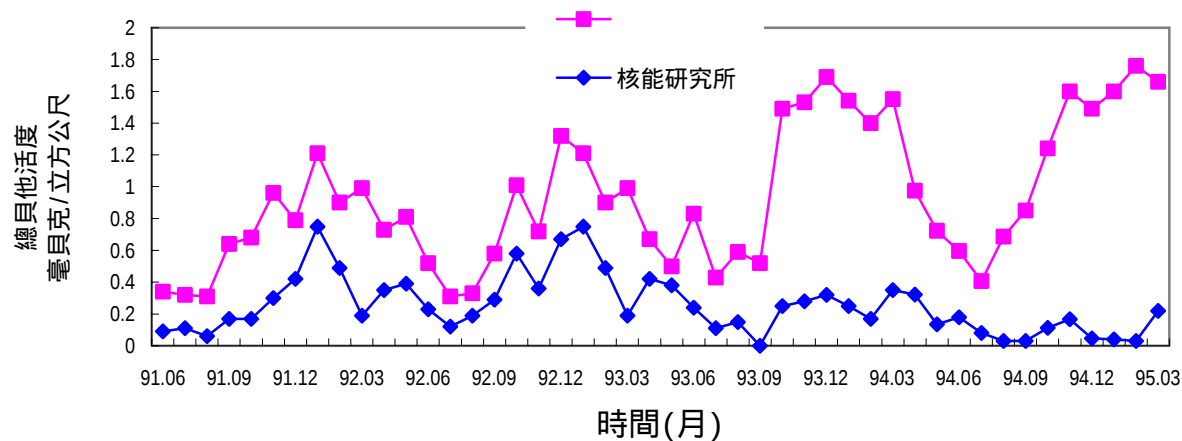
圖 2.18 研究用核設施周圍空浮微粒總貝他平均活度變動圖
